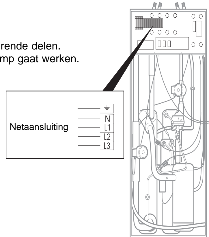
fig 5: Netaansluiting
