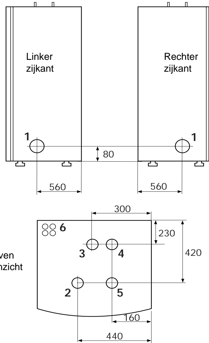
Fig. 4: Aansluit- en maatvoeringen
