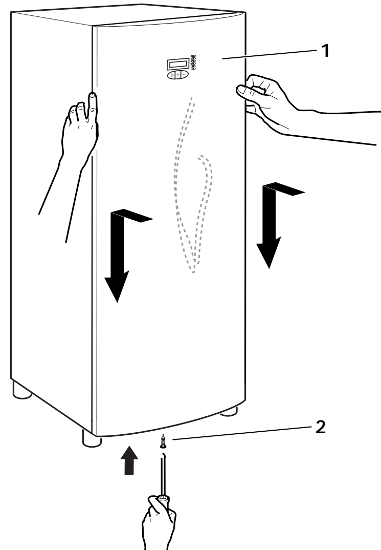
fig 14: Aanbrengen voorfront
