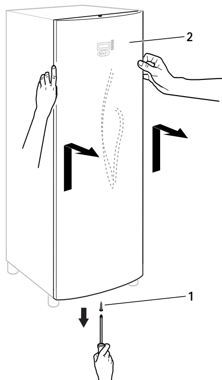
fig 2 frontplaat afnemen
