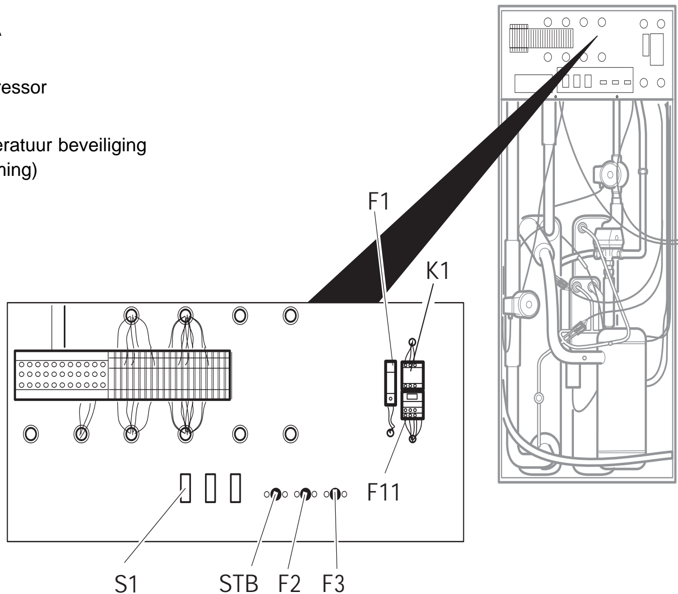
fig 11 :Lokatie van schakelaars en veiligheden
