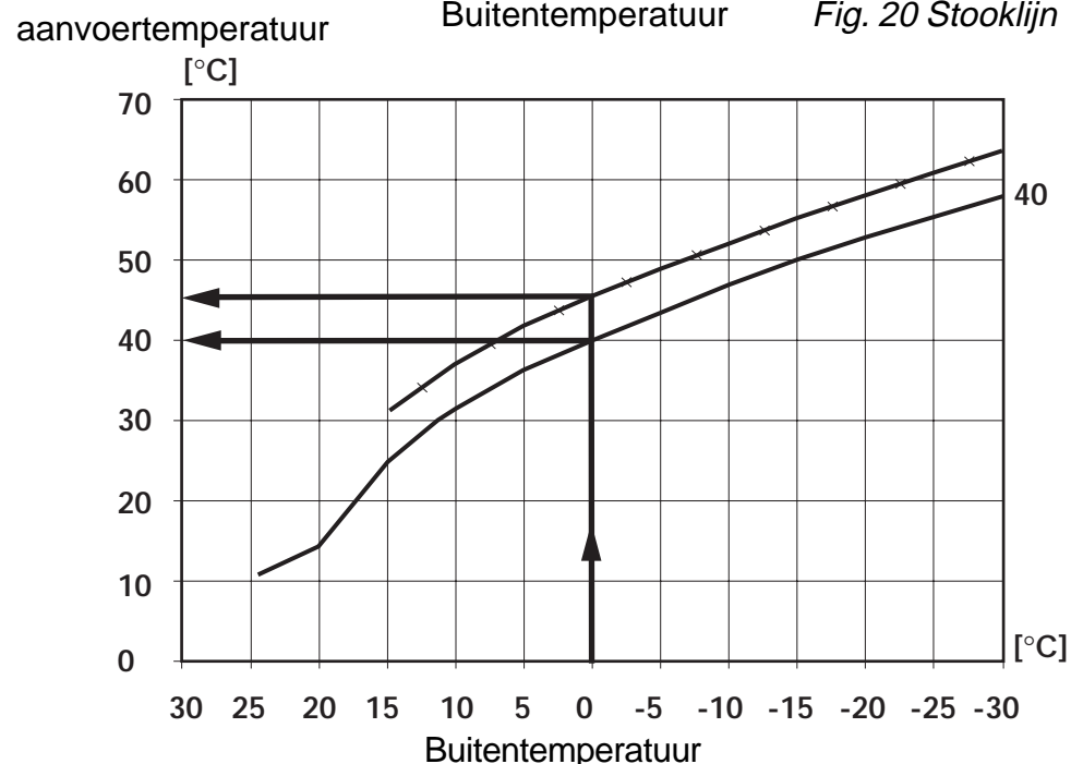
Fig. 21 Stooklijn verschuiving
