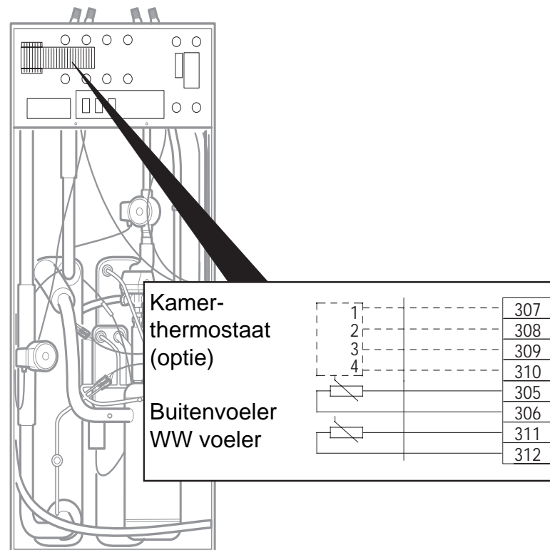
fig 6 :aansluitingen van regelapparatuur en externe voelers
