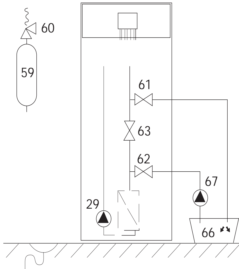
fig 12 :vullen van het brinesysteem
