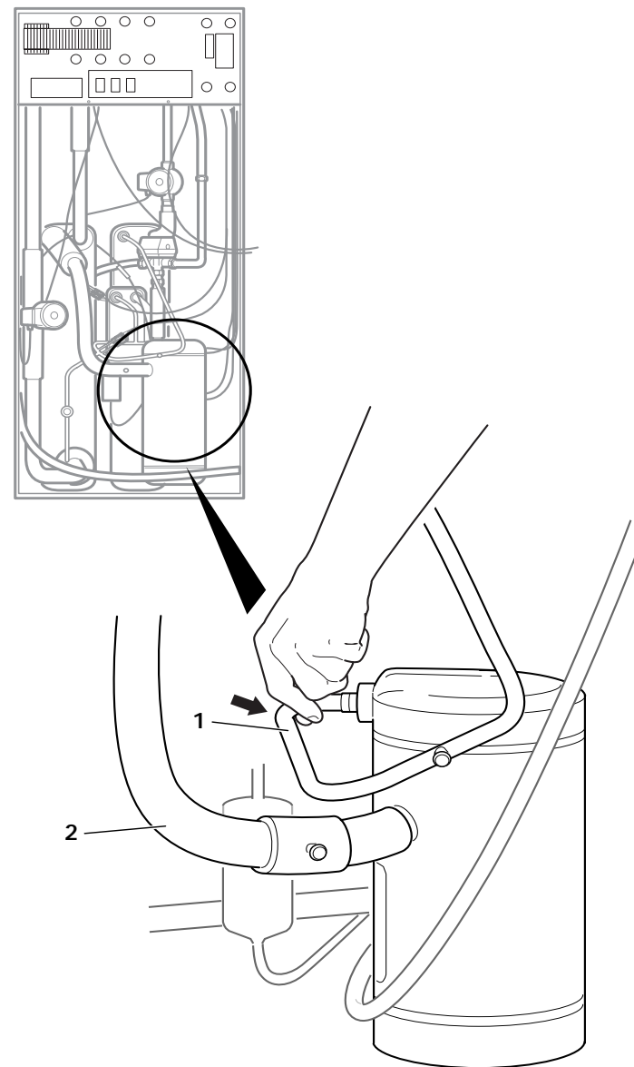
fig 13: Draairichting van de compressor controleren.
